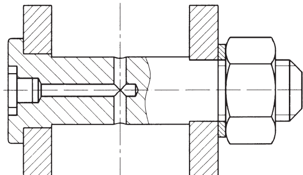
с гайкой или корончатой гайкой и шплинтом, смазочным ниппелем и смазочным отверстием
