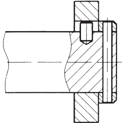
со стопорным кольцом, зажимной втулкой и стопорной шпилькой
