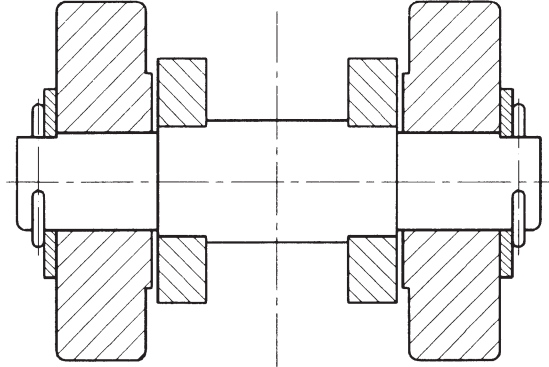
наружные ролики с шайбой и шплинтом
